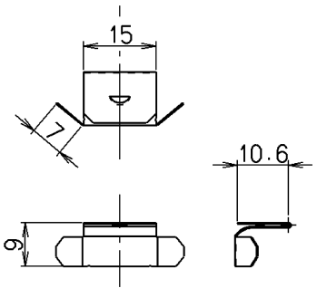
横幕板固定金具詳細 (S=1/1)
