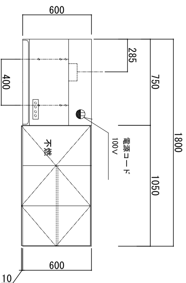
1412.5 水栓設置参考位置
