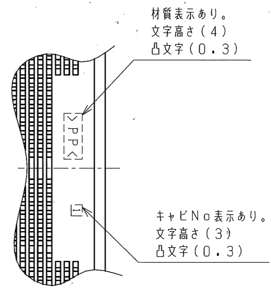
A矢視 (1:1)
