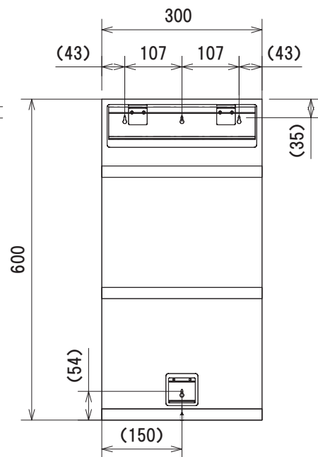
背面図S=1/10
