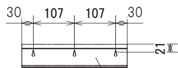
取付金具(上)
